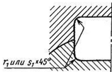
Шпоночные пазы вала и втулки
